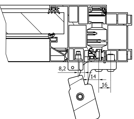
C ( 1:2 )
