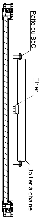
A-A ( 1:10 )
